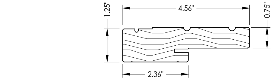
1 WOOD JAMB
